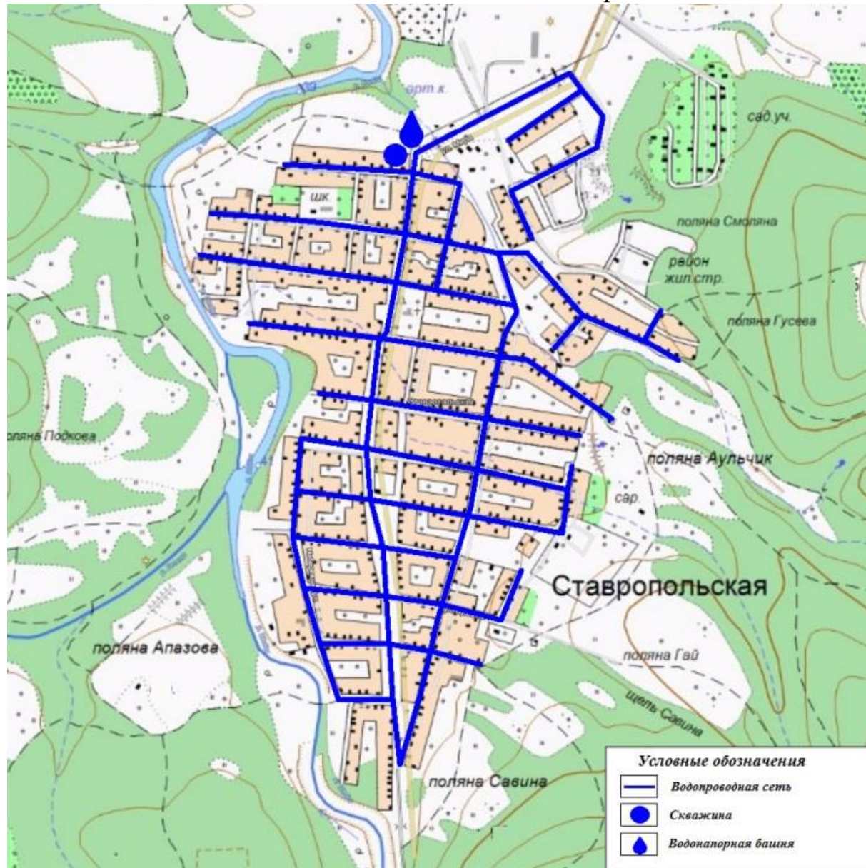
Схема водоснабжения ст. Ставропольская
