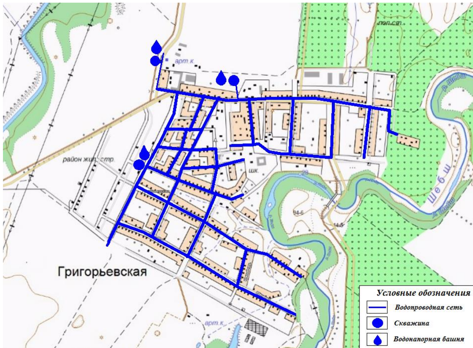
Схема водоснабжения ст. Григорьевская
